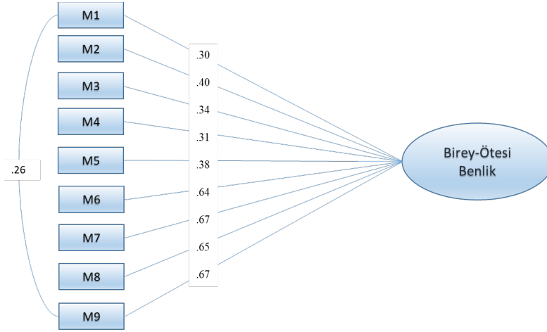
Şekil 1. Birey-Ötesi Benlik Ölçeği Faktör Yüklerini Gösterir Yol Diyagramı
